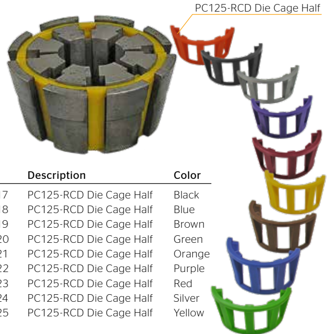
PC125-RCD Die Cage Half
